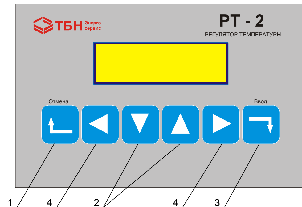
Рисунок 2а. Лицевая панель РТ-2 в отдельном исполнении.
