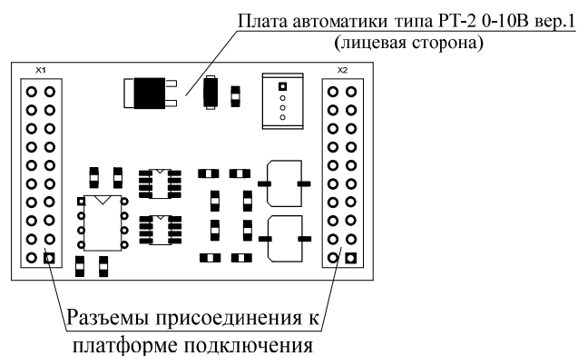
Рисунок 1 в. Обратная сторона платформы подключения и плата автоматики.
